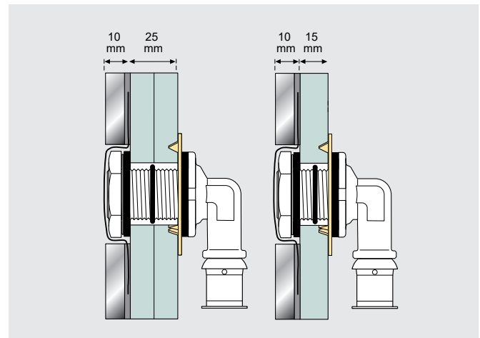
Proti-vrtenju zaščitena vgradnja v suhomontažno steno iz mavčnih plošč z Uponsor aretirnno ploščico LWC
