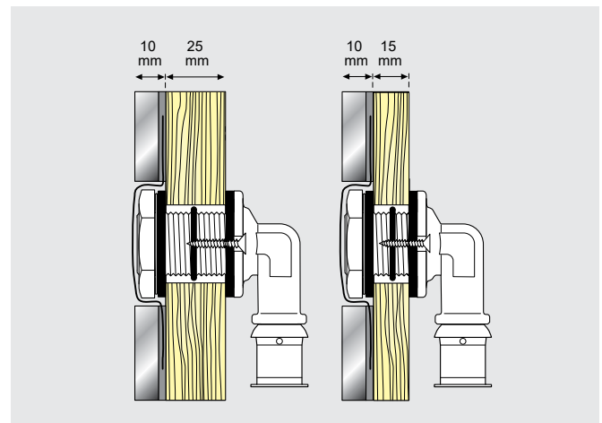
Proti-vrtenju zaščitena vgradnja v suhomontažno steno iz lesenih plošč z lesnimi vijaki, ki se dobijo na objektu
