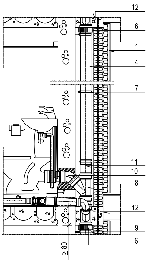
LEIKKAUS A-A
