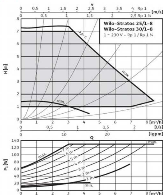
Δp-constant
