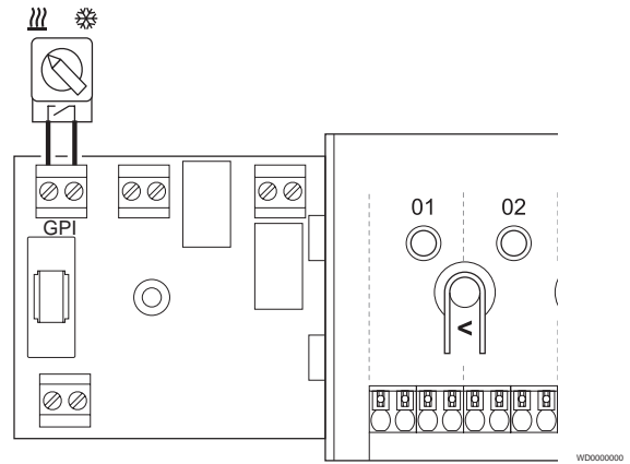
Vaihtokytkimen kytkentä pääkeskusyksikön GPI-liittimiin.
