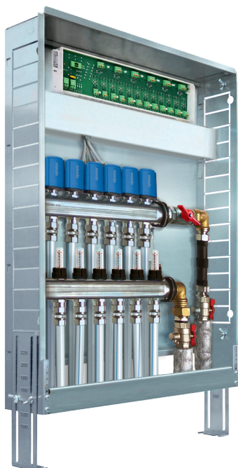
Uponor Base Flexiboard ermöglicht eine Vorverdrahtung ohne Belegungsplan in anschlussfertigen Verteilerstationen
