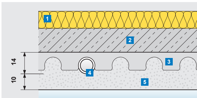
Shematski prikaz Uponorjevega Fix sistema na stropu
