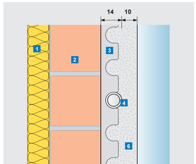
Shematski prikaz Uponorjevega Fix sistema na steni
