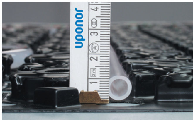
Samolepilna pritrdilna plošča minimalne višine
