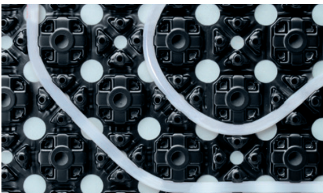
Vgradnja Uponor PE-Xa cevi pod kotom 45°
