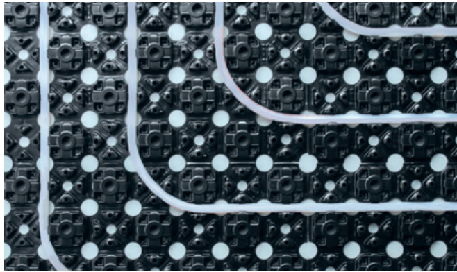
Vgradnja Uponor PE-Xa cevi pod kotom 90°
