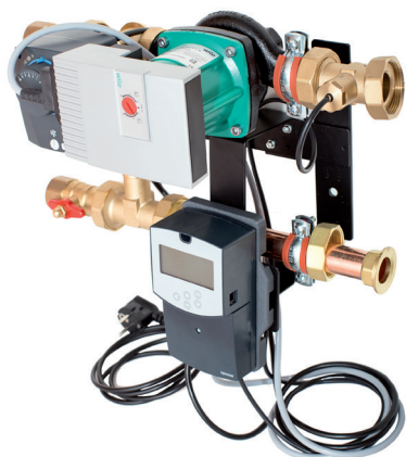
Bild: Uponor Fluvia Move Push PPG-30-A-W
