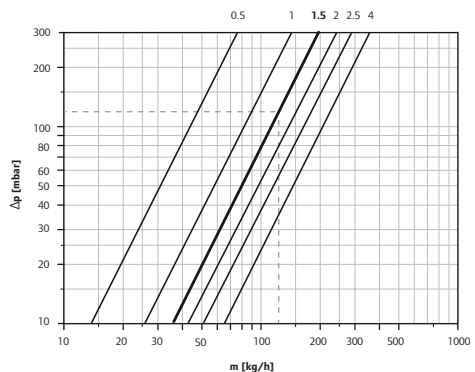
Bild: Differensstryck över ventil, två-rörssystemutförande.
