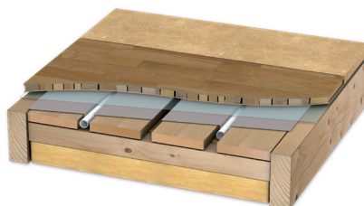
Bild: I träbjälklag
