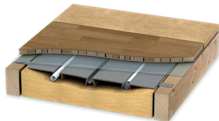
Bild: Golvvärmekassett utan isolering
