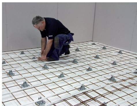
5. När röret är fäst i vändningarna går det lätt och snabbt att naja hela installationen.
