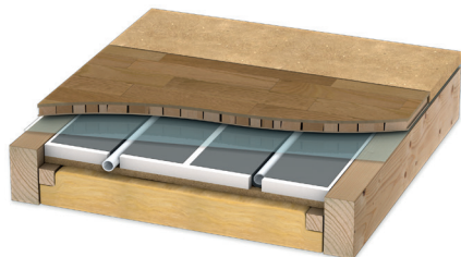
Bild: Golvvärmekassett med isolering
