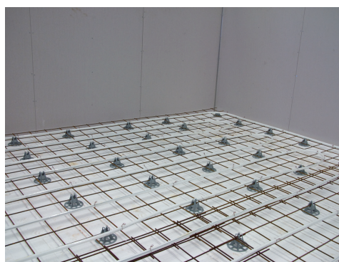
7. Täck rörens hjässa med minst 30 mm betong för att säkerhetsställa värmespridning.
