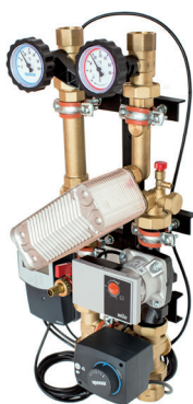
Bild: Uponor Fluvia Move Push EPG-6-A-W
