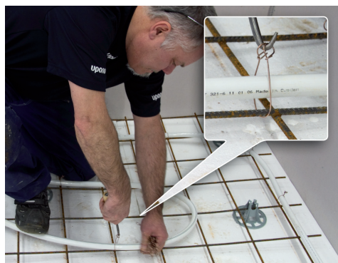
3. Naja fast röret i vändningarna
