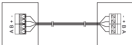
Bild: Termostat och reglercentral
