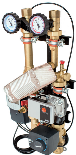
Bild: Uponor Fluvia Move Push EPG-6-A-W
