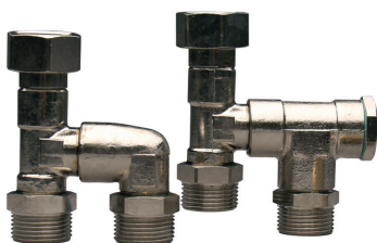
Bild: Grenrör för två slingor
