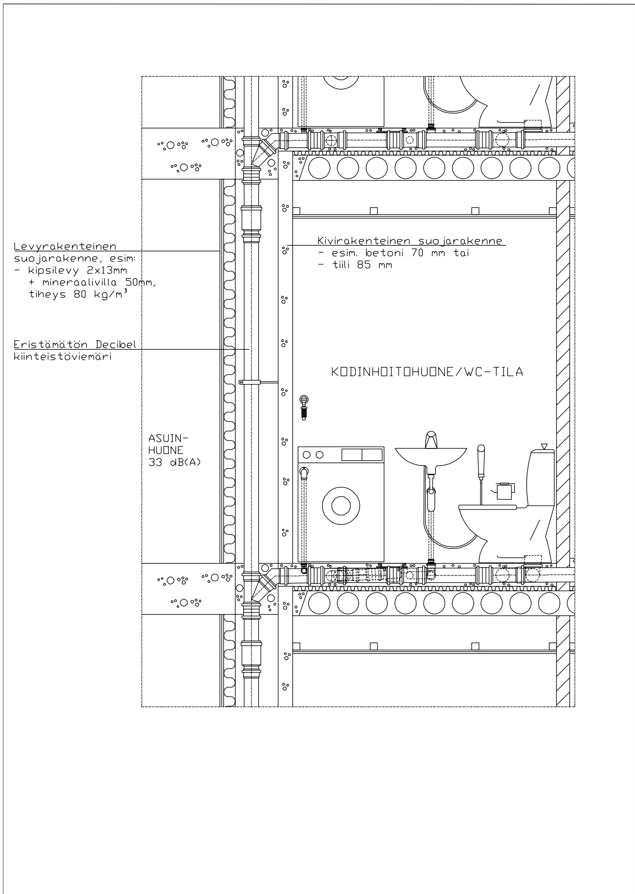
KUVA 7. Eristämättömän Uponor Decibel -kiinteistöviemäriin äänitekniset suojarakenteet, äänitasovaatimus 33 dB(A). Mikäli suojarakenteen rakenteet ovat kevyitä, viemäriputki kannakoidaan kerrosten välillä tärinäneristimiä hyödyntäen. EI 30.
