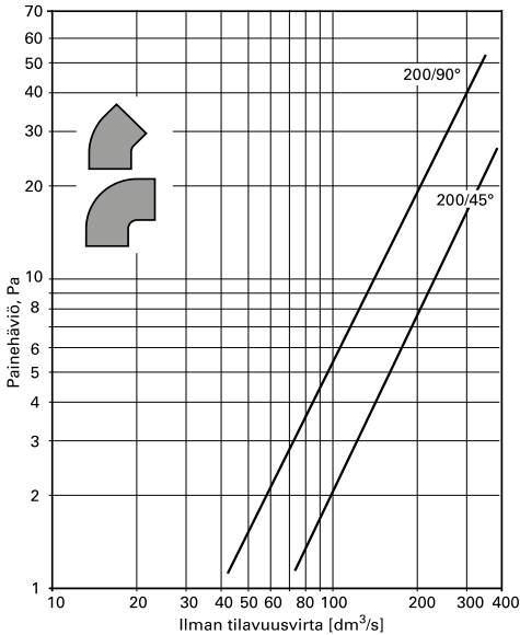
Käyrät 200/45° ja 200/90°
