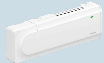
Keskusyksikkö Smatrx Wave Pulse Yksi keskusyksikkö voi ohjata 6 termostaattia ja 8 toimilaitetta LVI-nro 2988495
