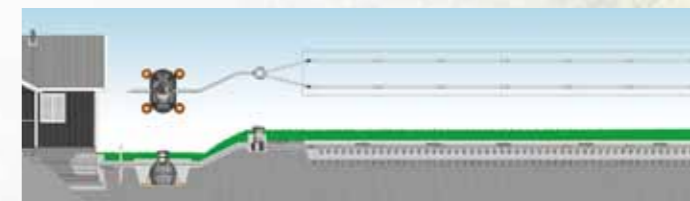
2 m 3 septiņš ar sūkni un infiltrācijas sistēmu (Uponor-No 321013)
