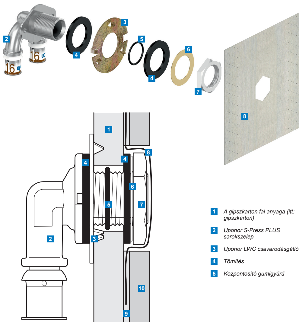
Szakszerűen tömitett Uponor S-Press PLUS U LWC könyök fal tömitőgyűrű Uponor LWC szerelőkészlettel és Uponor LWC tömitőperemmel
