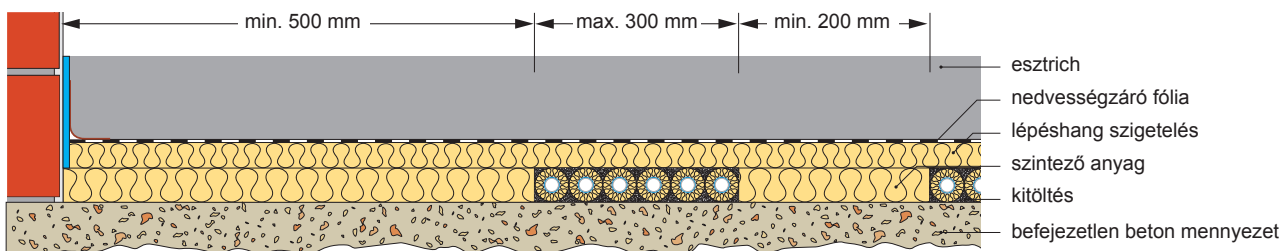
Távolság a faltól a csőig/csővezeték nyomvonaláig, beleértve a szigetelést és az esztrichet a folyosókon kívüli helyiségekben
