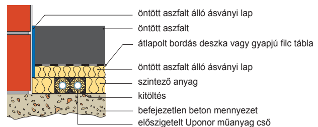
Padló szerkezet öntött aszfalttal
