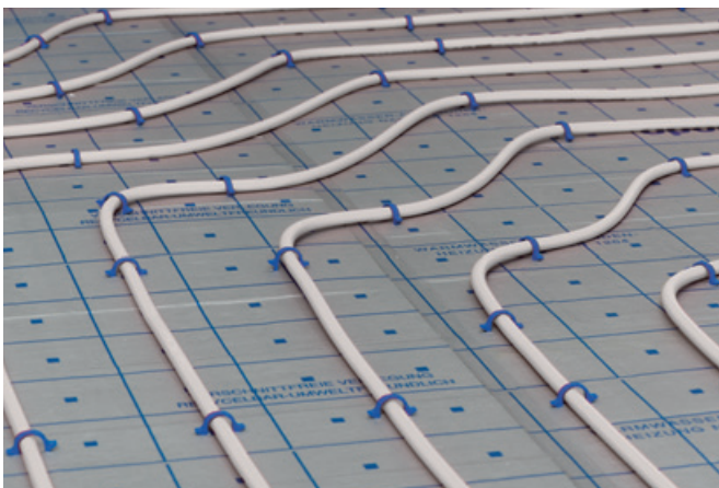
Enoten in jasen vzorec polaganja cevi zahvaljujoč natiskani mreži in čvrstim pritrdilci
