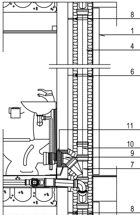
LEIKKAUS A-A
