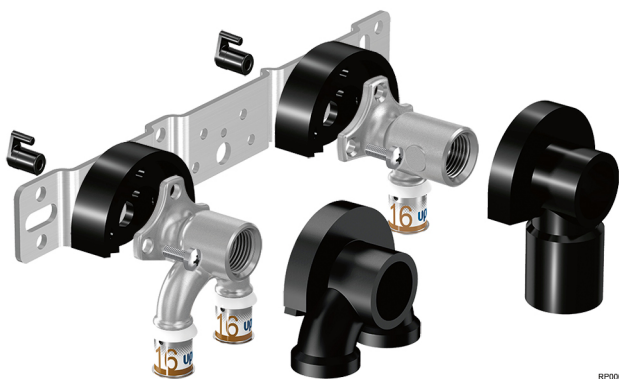
Uponor S-Press PLUS U-veggbraketter med redusert tilkobling på den ene siden
