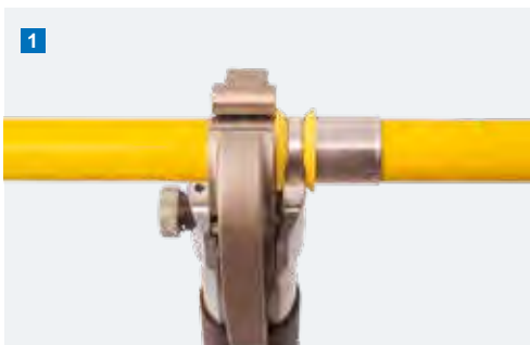
1 Persbek tegen de gele persbek- geleiding van de pershuls leggen
