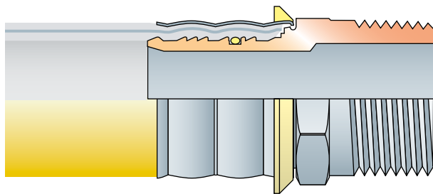
Doorsnedetekening Uponor GAS Press persfitting met RVS-pershuls
