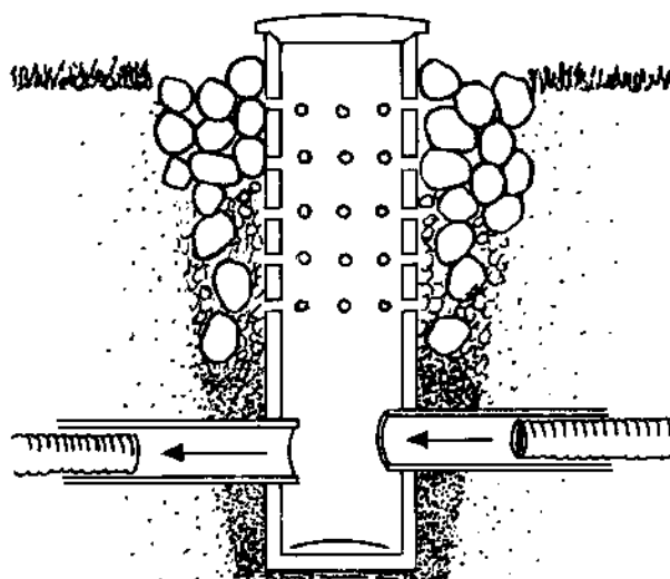
Ytvattenbrunn/kopplingsbrunn
