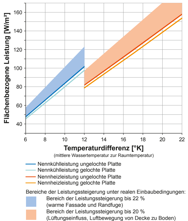
Heiz-/Kühlleistung Uponor Thermatop M, geprüft nach DIN EN 14240 bzw. DIN EN 14037
