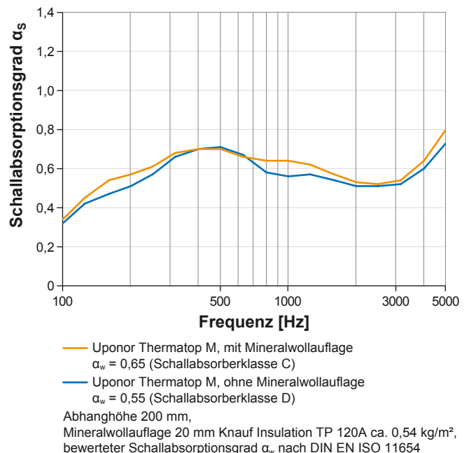
Schallabsorption Uponor Thermatop M, geprüft nach DIN EN ISO 354
