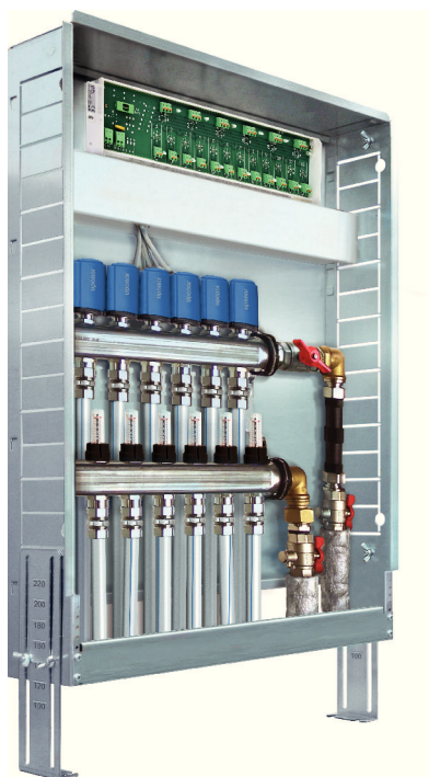
„Flexiboard“ montavimo kolektorinėse spintelėse pavyzdys
