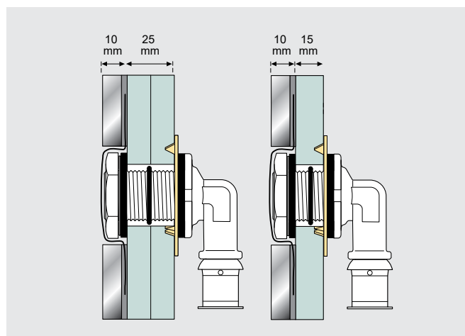
Proti-vrtenju zaščiten vgradnja v suhomontažno steno iz mavčnih plošč z Uponsor aretira ploščico LWC
