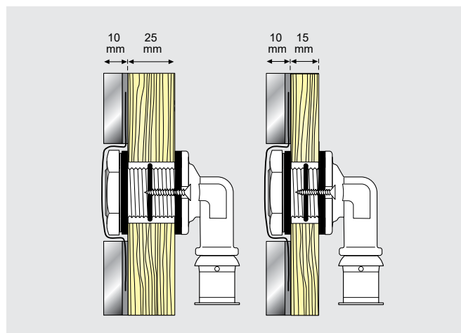
Proti-vrtenju zaščiten vgradnja v suhomontažno steno iz lesenih plošč z lesnimi vijaki, ki se dobijo na objektu
