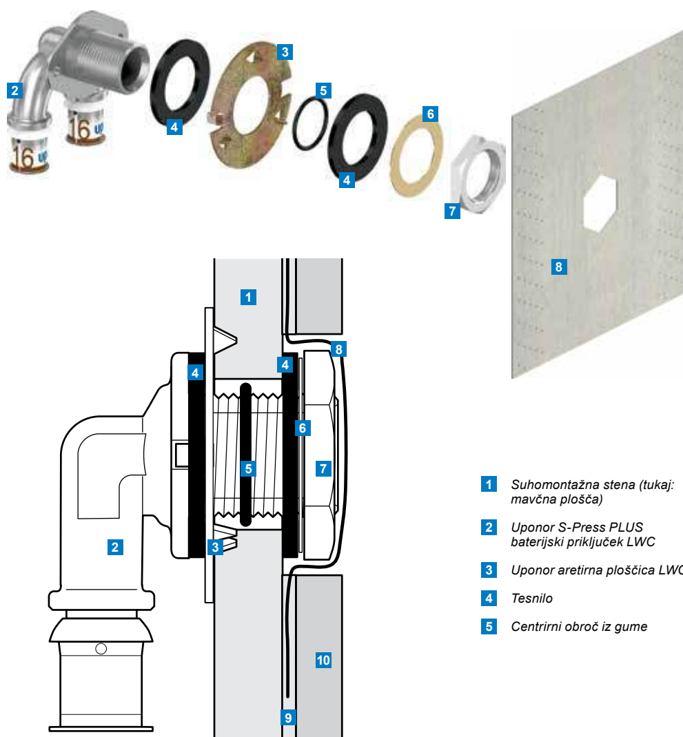
Profesionalno zatesnjen kotni Uponor U-baterijski priključek LWC z Uponor LWC montažnim in tesnilnim setom
