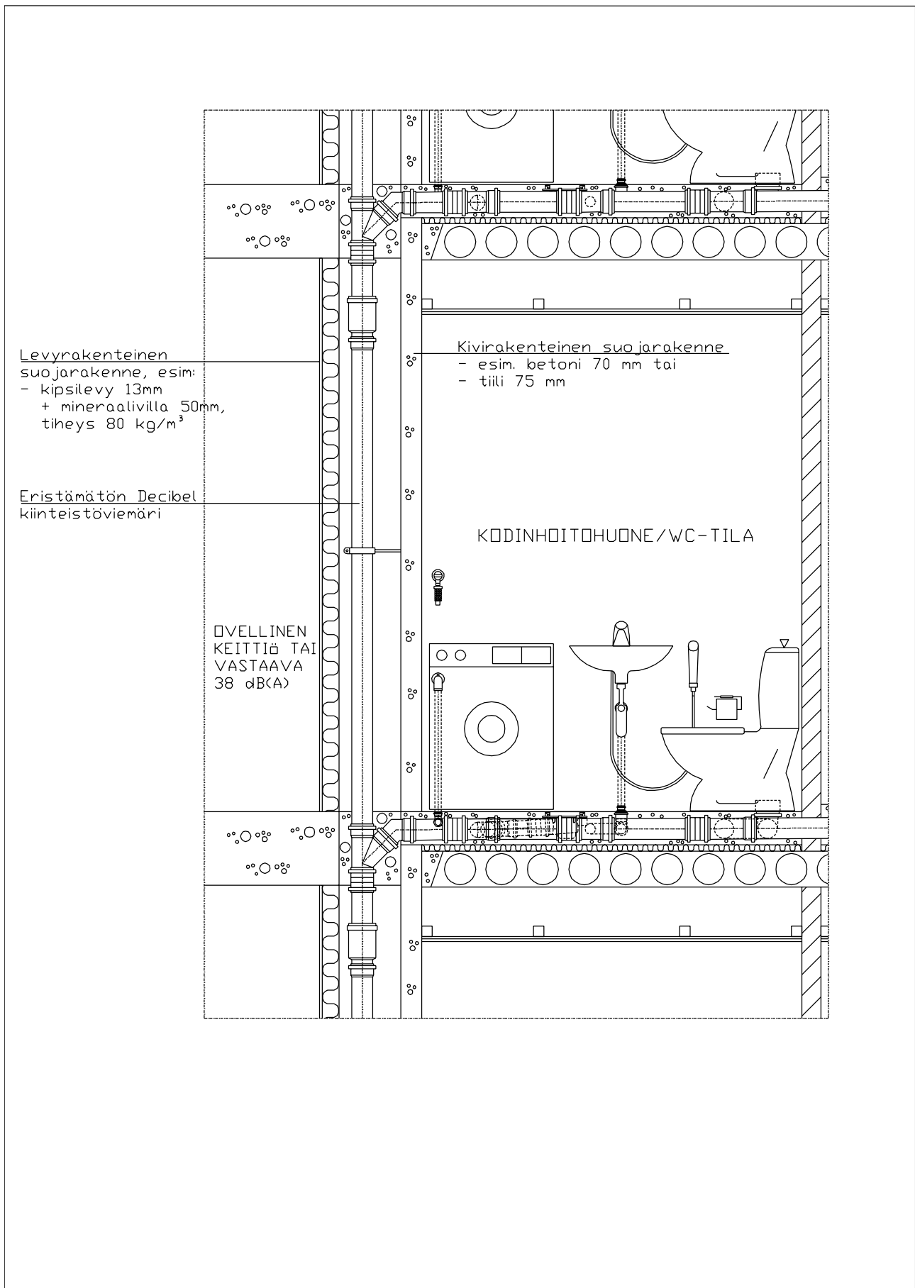
KUVA 6. Eristämättömän Uponor Decibel -kiinteistöviemärin äänitekniset suojarakenteet, äänitasovaatimus 38 dB(A). Mikäli suojarakenteen rakenteet ovat kevyitä, viemäriputki kannakoidaan kerrosten välillä tärinäneristimiä hyödyntäen. EI 30.
