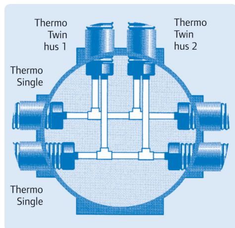
Bild 49: Värmeförsörjning från huvudledningen till två hus
