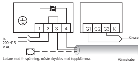
Bild: Matningens, värmekabelns och givarens ledningsdragnig
