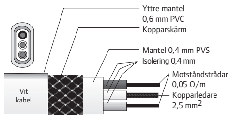
Bild: 230 V/400 V, 2x0,05 Ω/m (min. 150 - max. 700 m)
