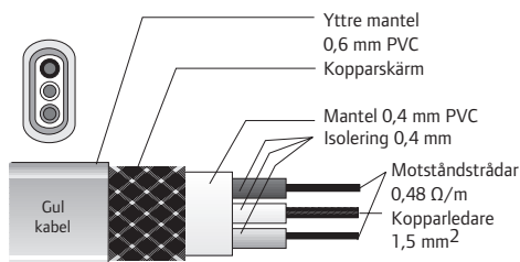
Bild: 230 V/400 V, 2x0,48 Ω/m (min. 50 - max. 300 m)
