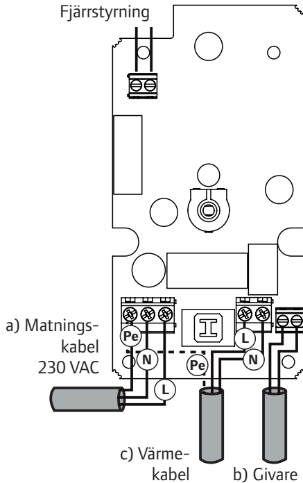
Bild: Kopplingsschema styrenhet
