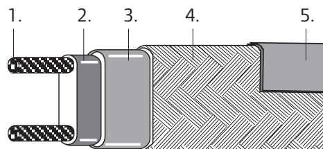
Bild: Självreglerande värmekabel, genomskärning
