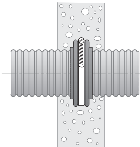
Bild: Ingjutningsring i betongvägg
