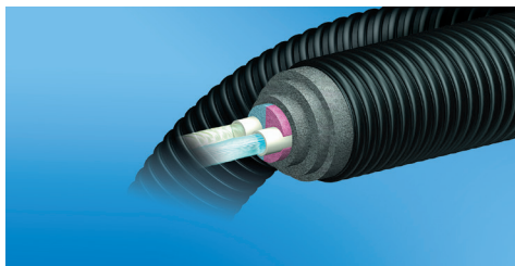
Bild: Uponor Ecoflex Aqua Twin
