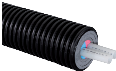
Bild: Uponor Ecoflex Thermo Twin
