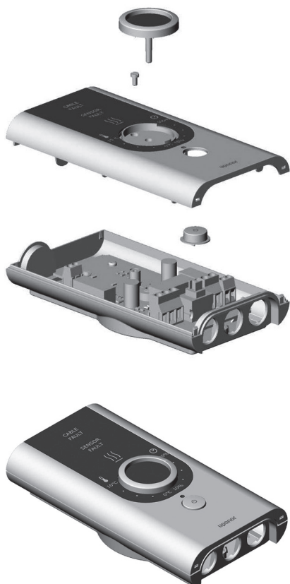
Bild: Montering av styrenheten
