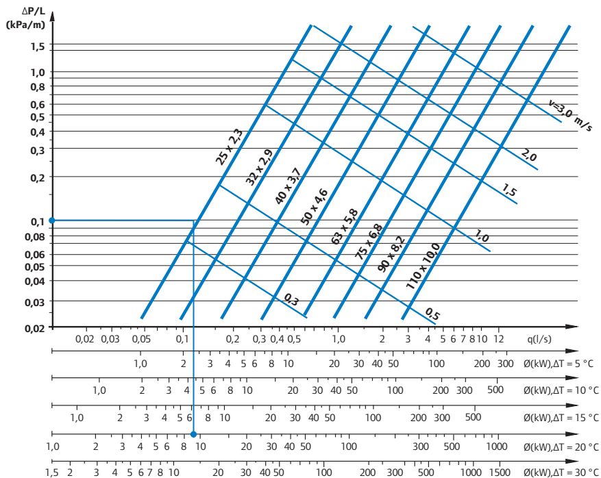
Bild: Effektvården vid temperaturskillnader
