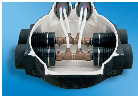
Bild: Kopplingsbrunn, genomskäring
