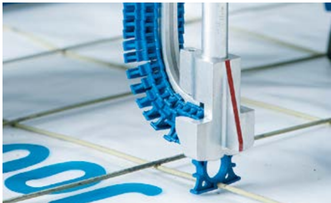
Brzo, precizno i otporno pričvršćivanje: Uponor Classic Clipmaster čvrsto drži pričvrsnice Uponor Classic Master i osigurava savršeno postavljanje
