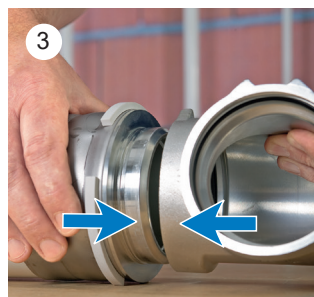
Kuva 1. Asenna viistetty komposiittiputki Uponor RS-liitinjärjestelmän puristuspaahan.
