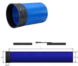
Ø600-1000:
